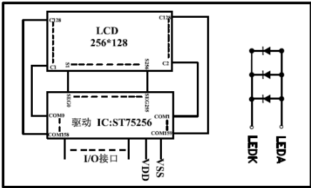
电路框图
