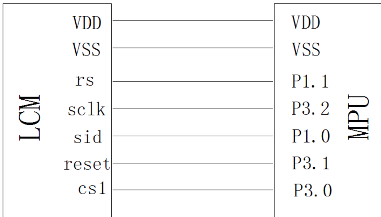
图 4. 串行接口
