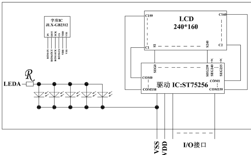
图 2: JLX240160G-676-PC 电路框图
