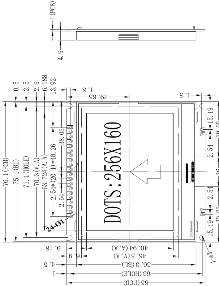
正面图
