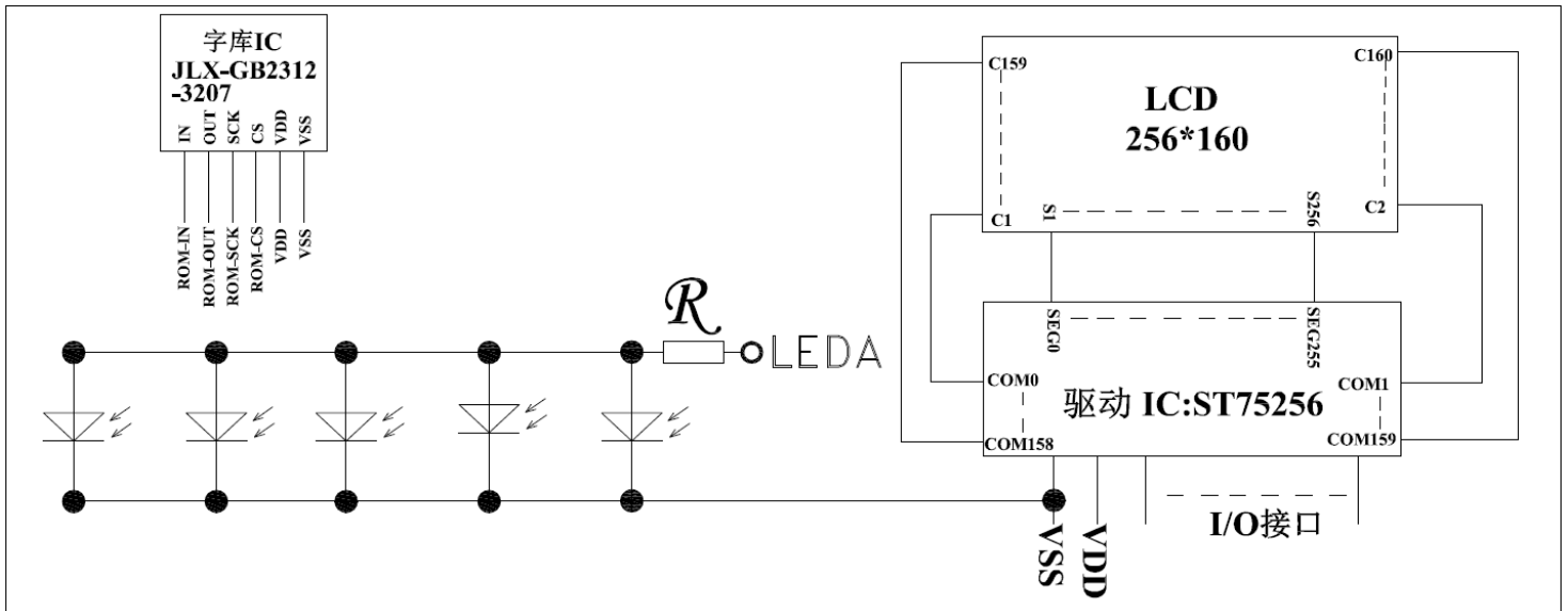
图 2: JLX256160G-910-PL 电路框图
