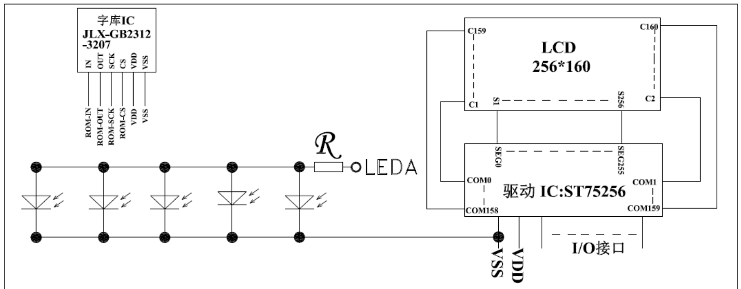
图 2: JLX256160G-91002-PL 电路框图
