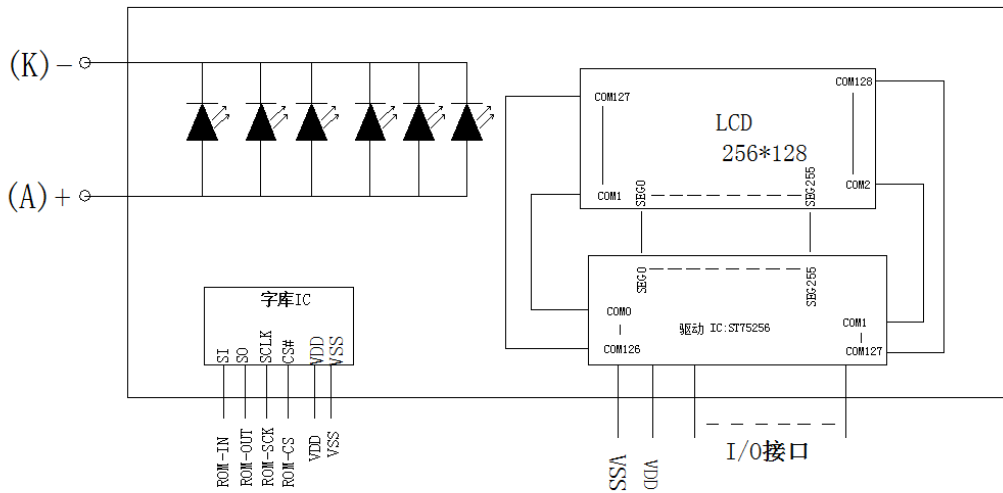
图 2: JLX256128G-931-PL 电路框图
