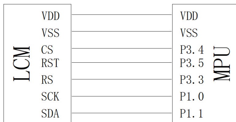
图 9. 串行接口
