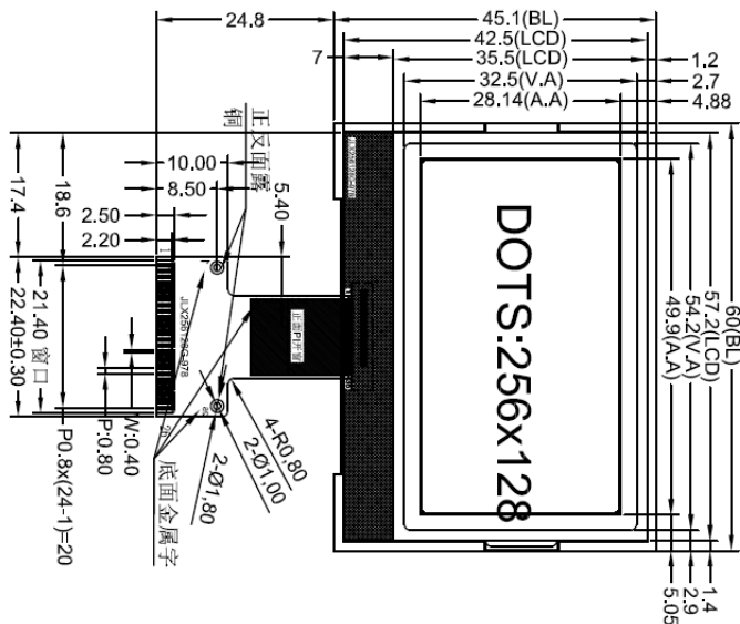
正面图
