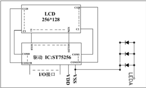
电路框图
