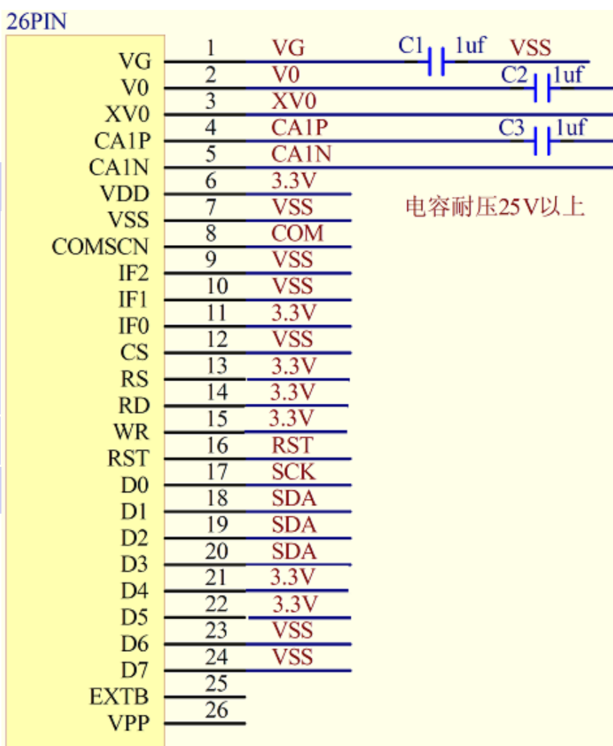
图 10. IIC
