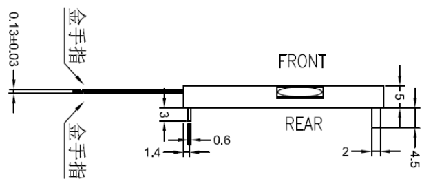
侧面图
