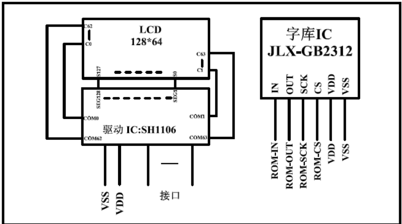
图 2: JLX12864OLED-13001-PC
