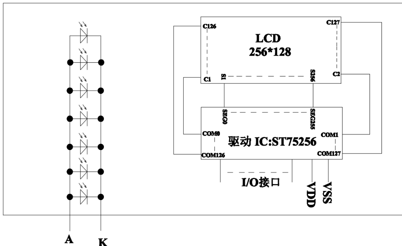
图 2: JLX256128G-975 图像点阵型液晶模块的电路框图
