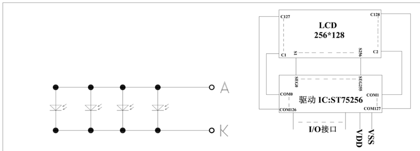
图 2:JLX256128G-92006-BN 图像点阵型液晶模块的电路框图
