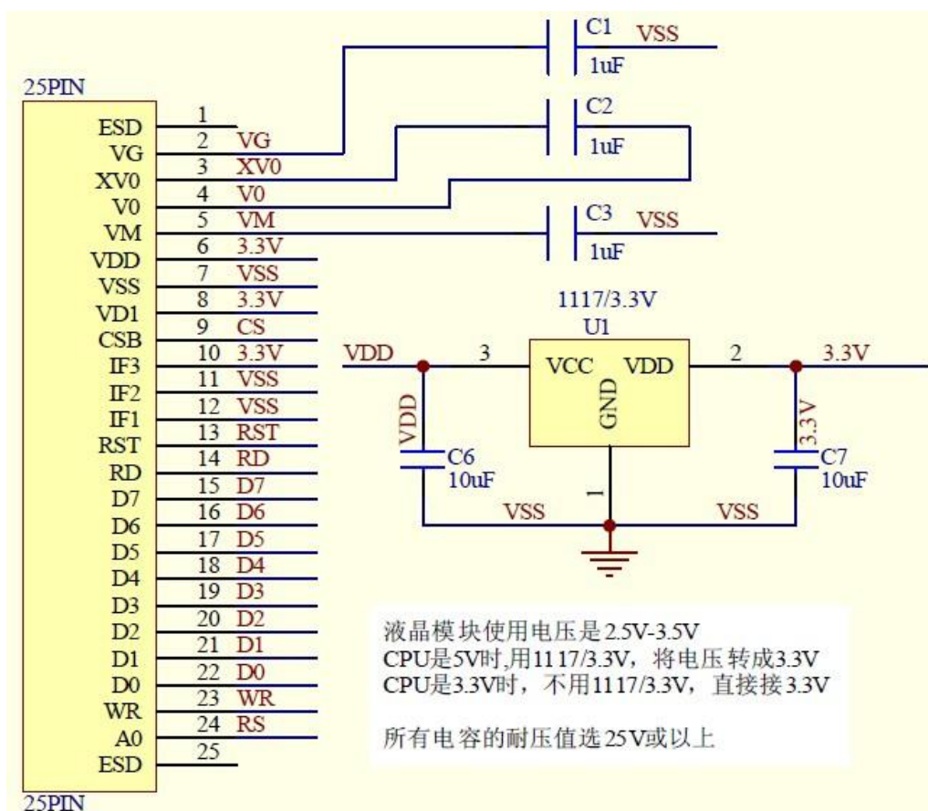
并行接口图
