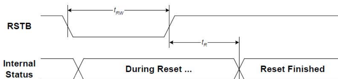
图 7：电源启动后复位的时序
