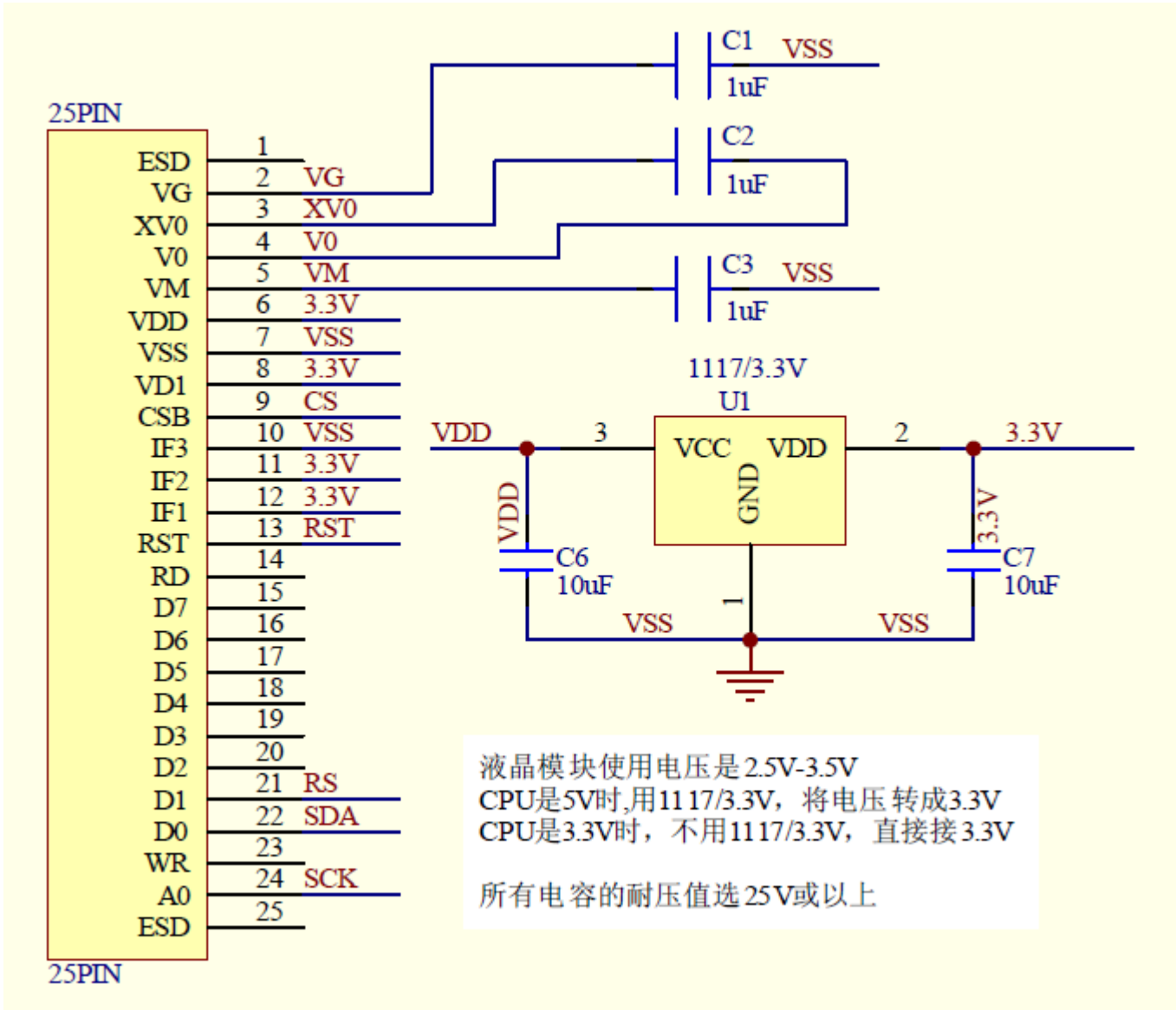
图 9. 串行接口
