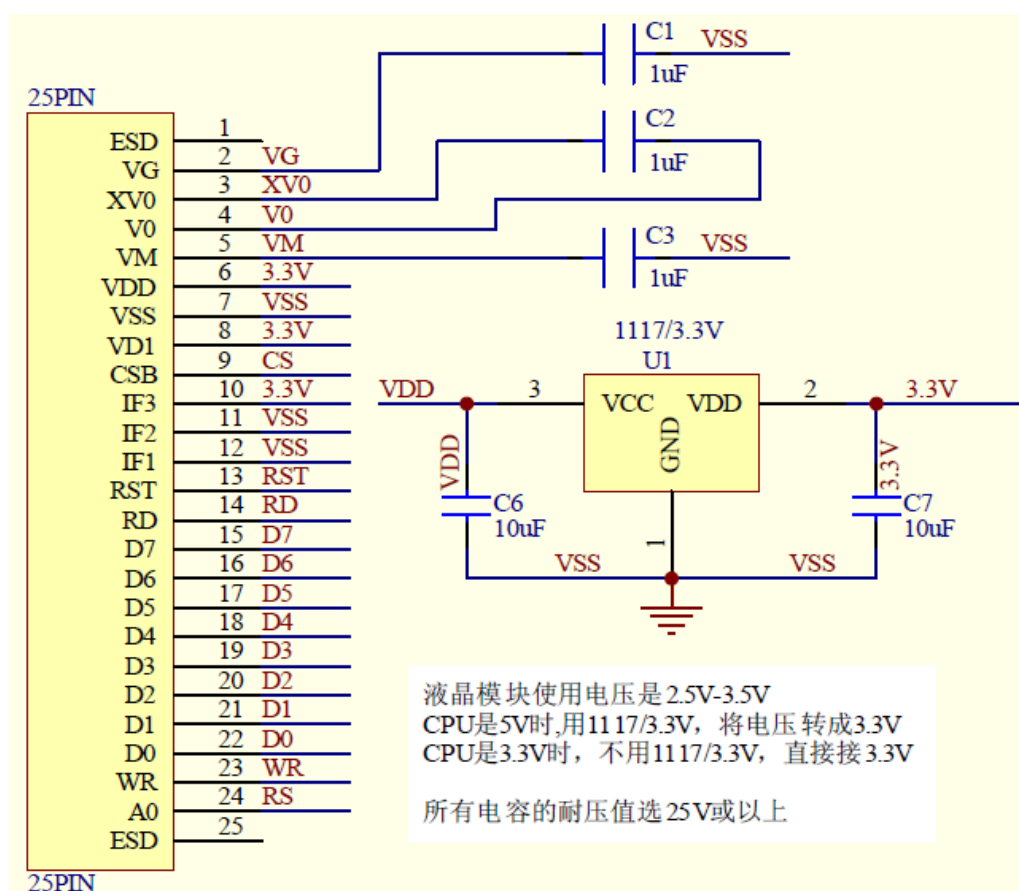
并行接口图
