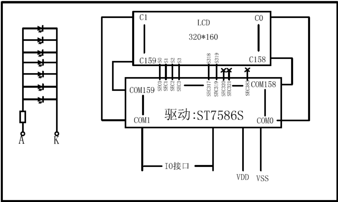
图 2: JLX320160G-969-BN 图像点阵型液晶模块的电路框图
