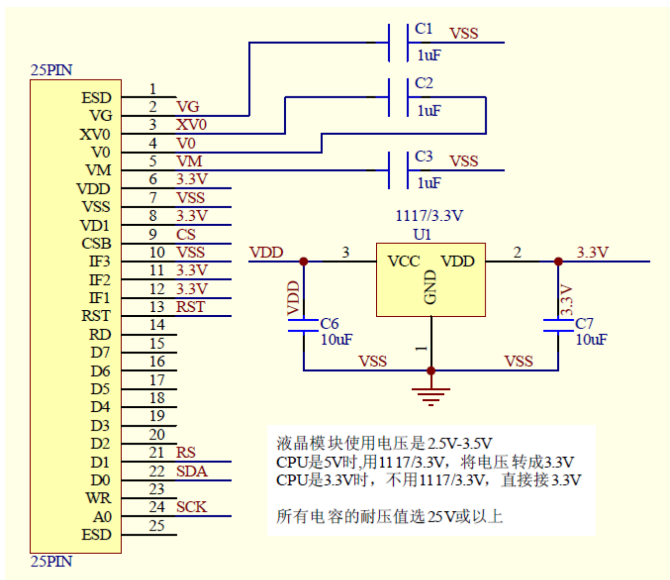
图 9. 串行接口
