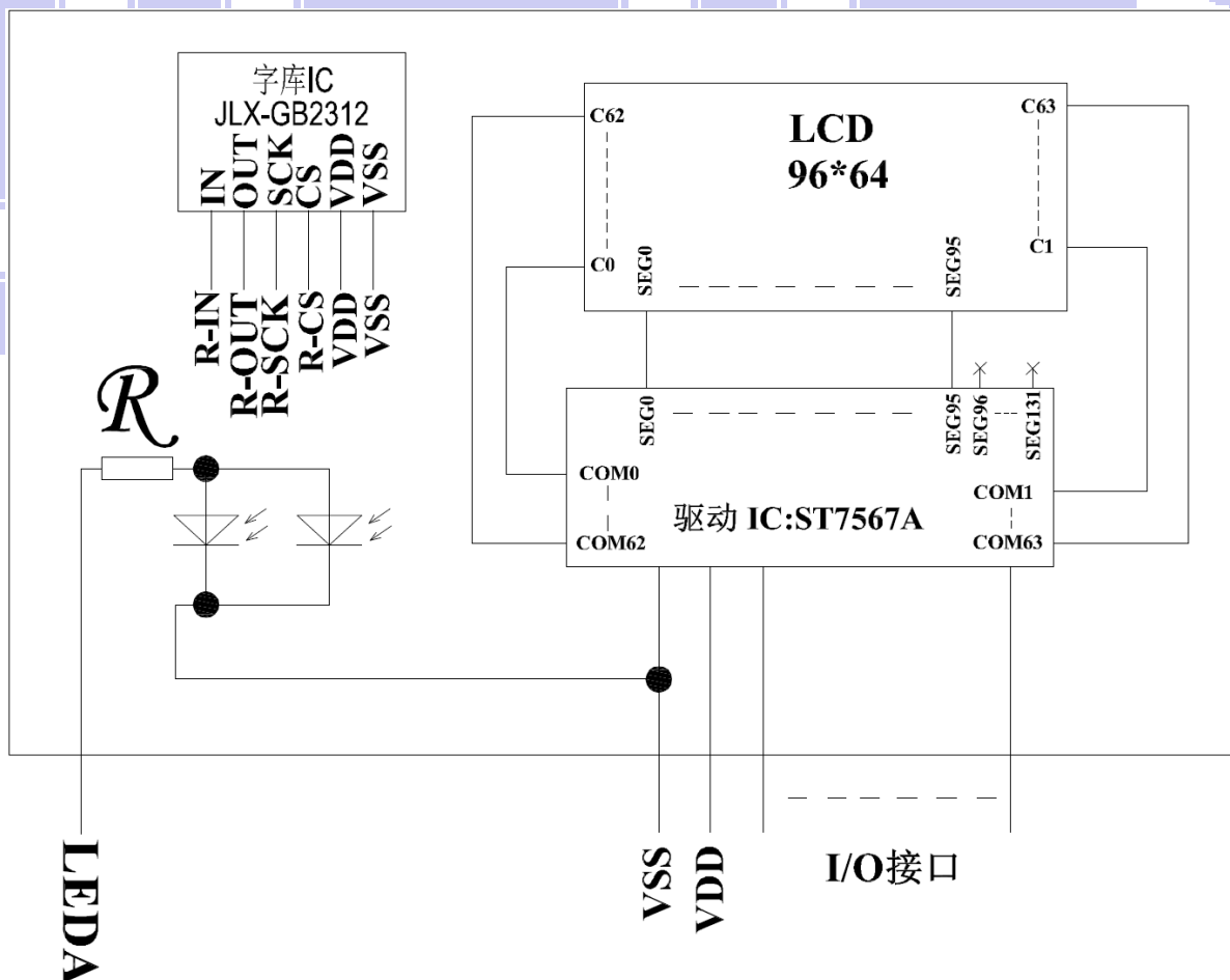
图 2: JLX9664G-959 图像点阵型液晶模块的电路框图
