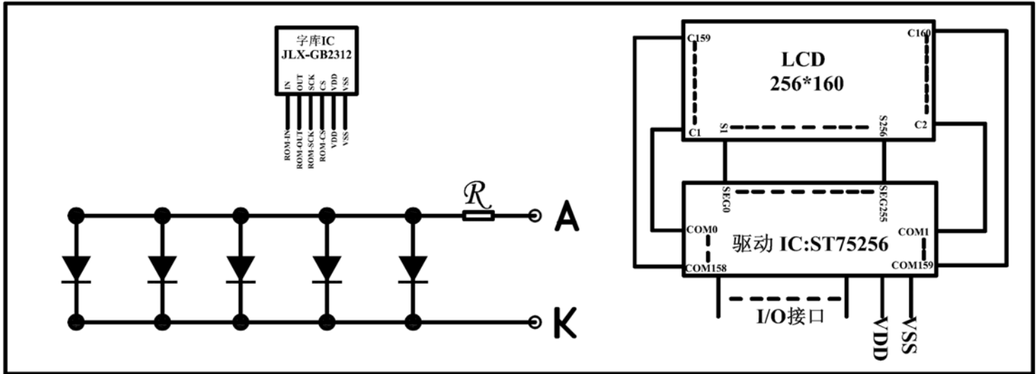
图 2: JLX256160G-910-PL 电路框图
