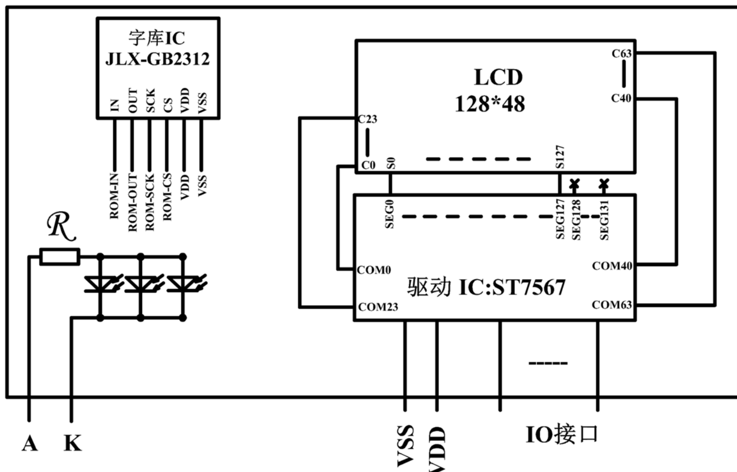
图 2: JLX12848G-942 电路框图
