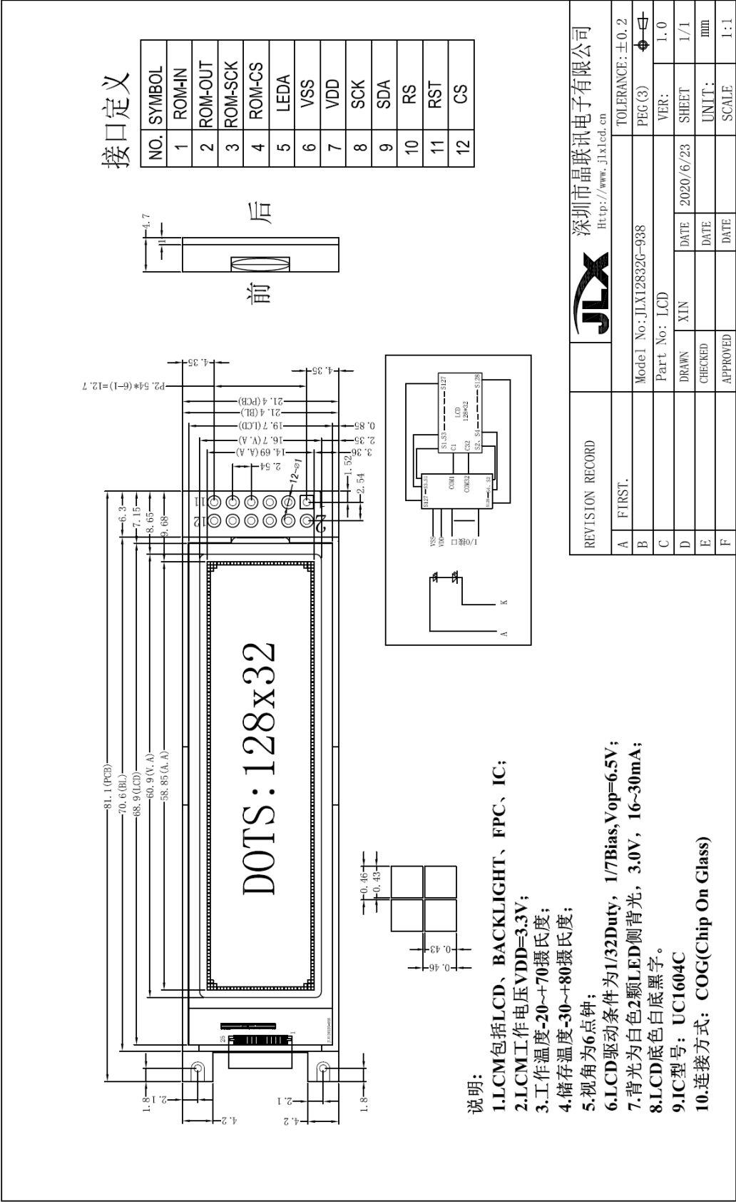
图 1. 外形尺寸
