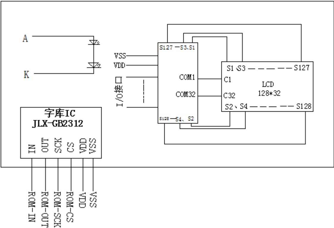
图 2: 电路框图
