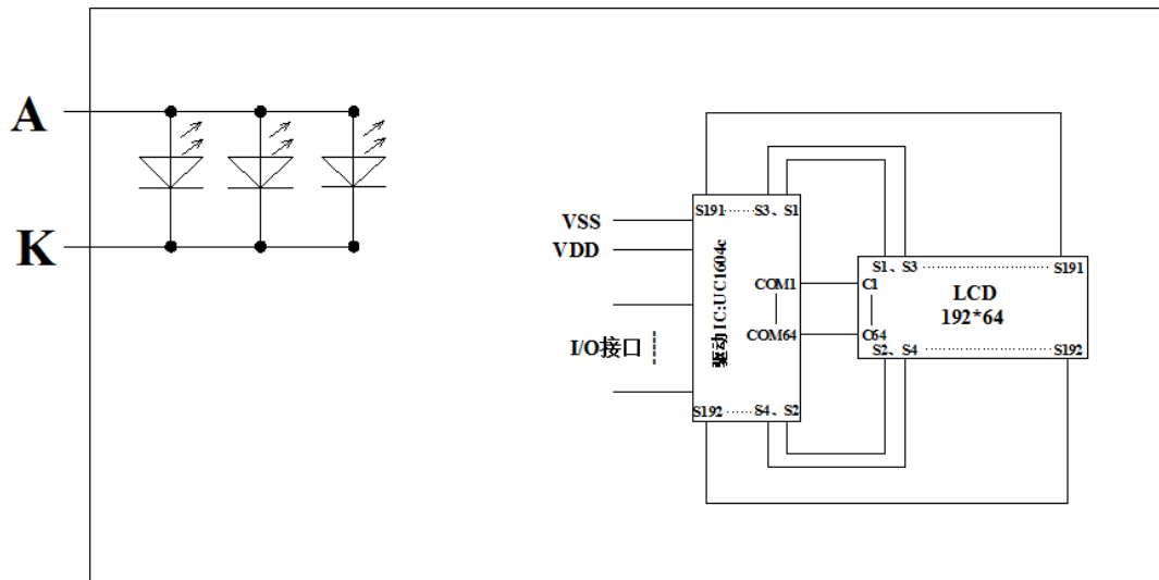
图 2: JLX19264G-26006 图像点阵型液晶模块的电路框图
