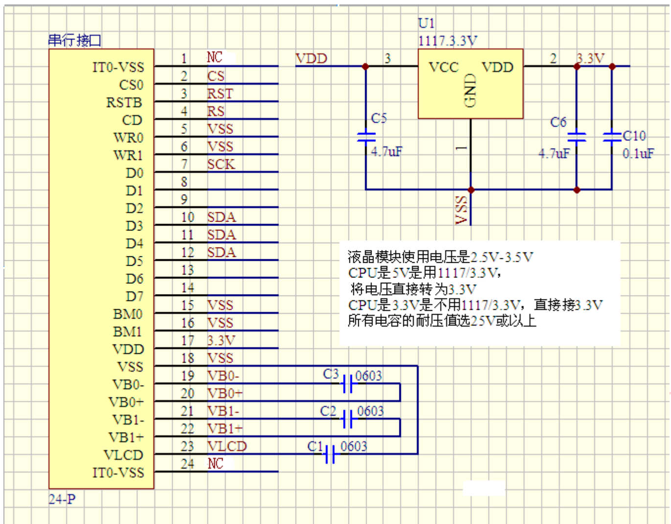
串行电路图
