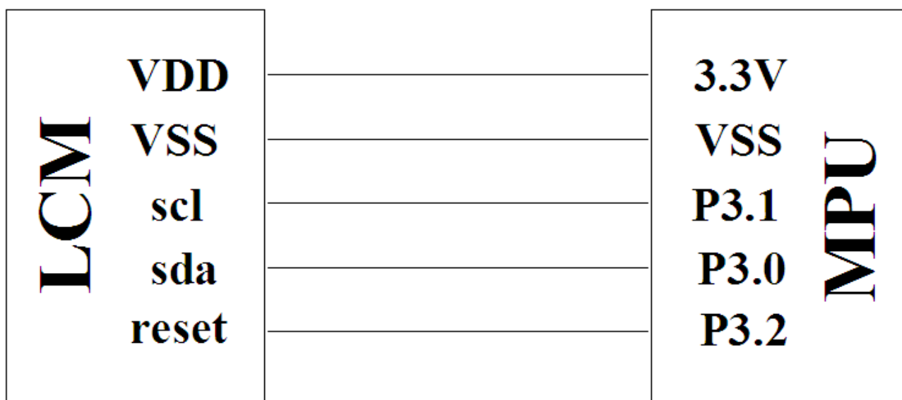
图 9. IIC 接口
