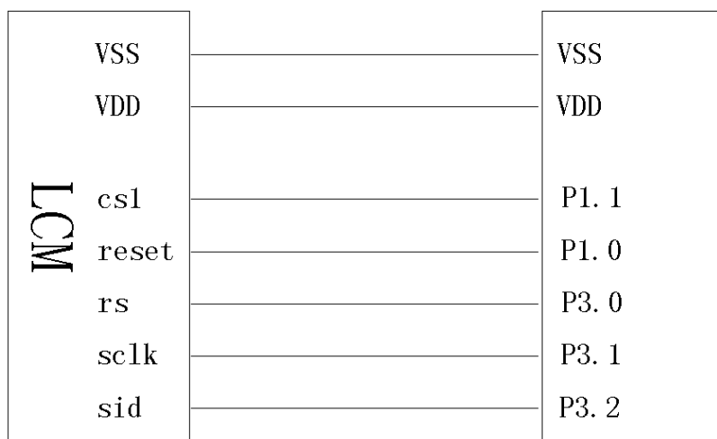
图 8. 串行接口
