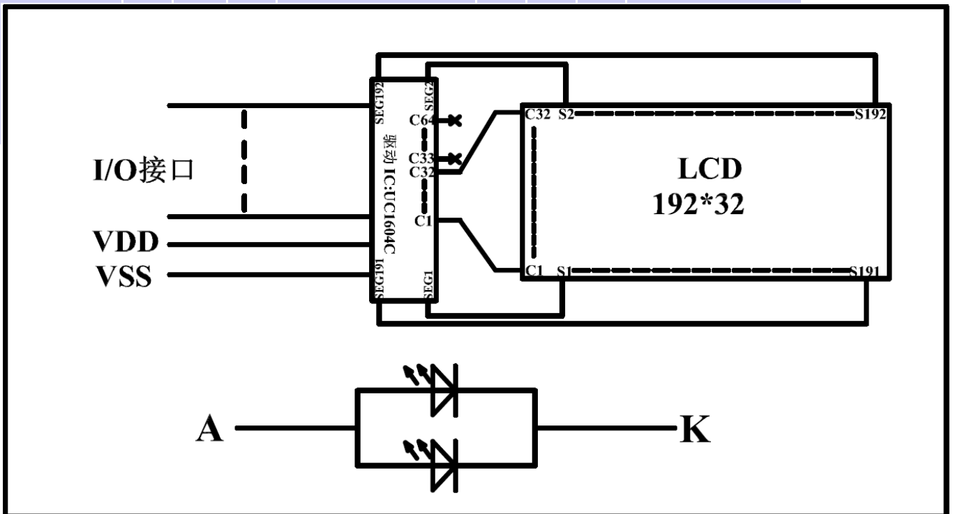
图 2: JLX19232G-927 图像点阵型液晶模块的电路框图
