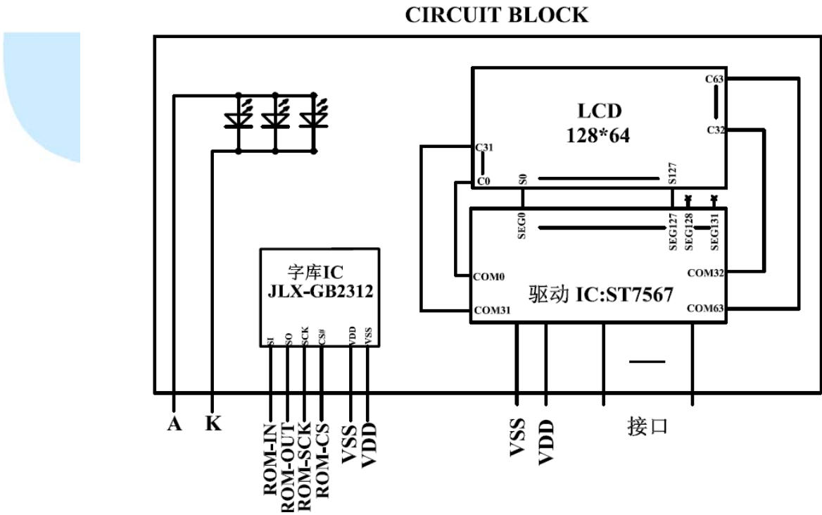
图 2: 电路框图
