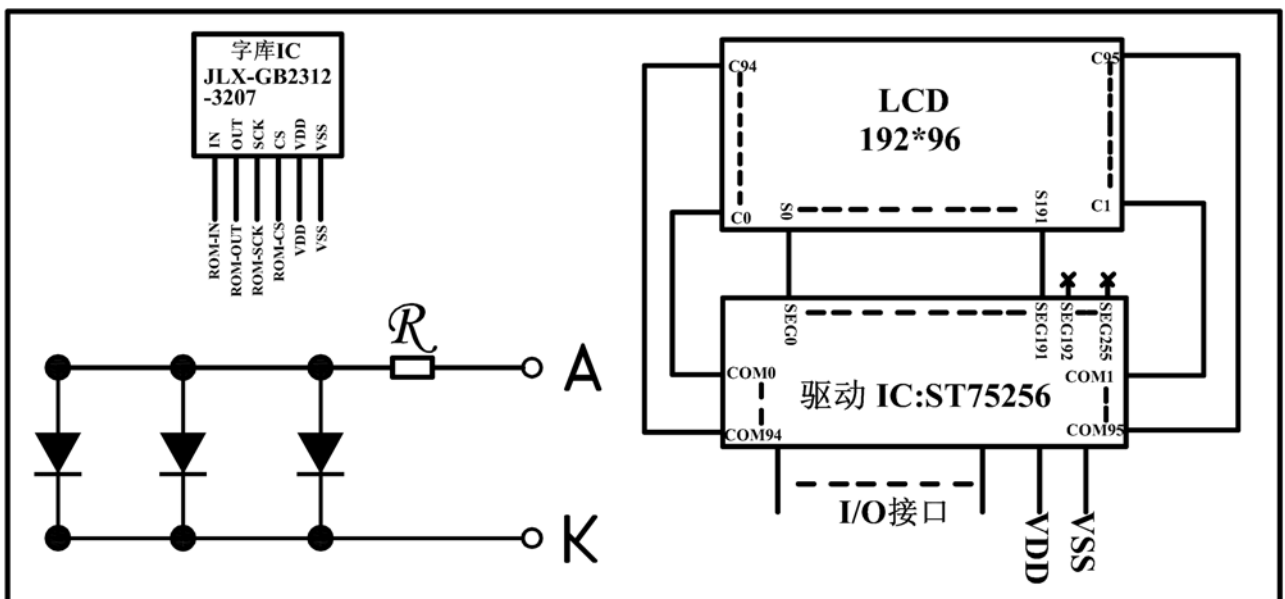
图 2: JLX19296G-909 电路框图
