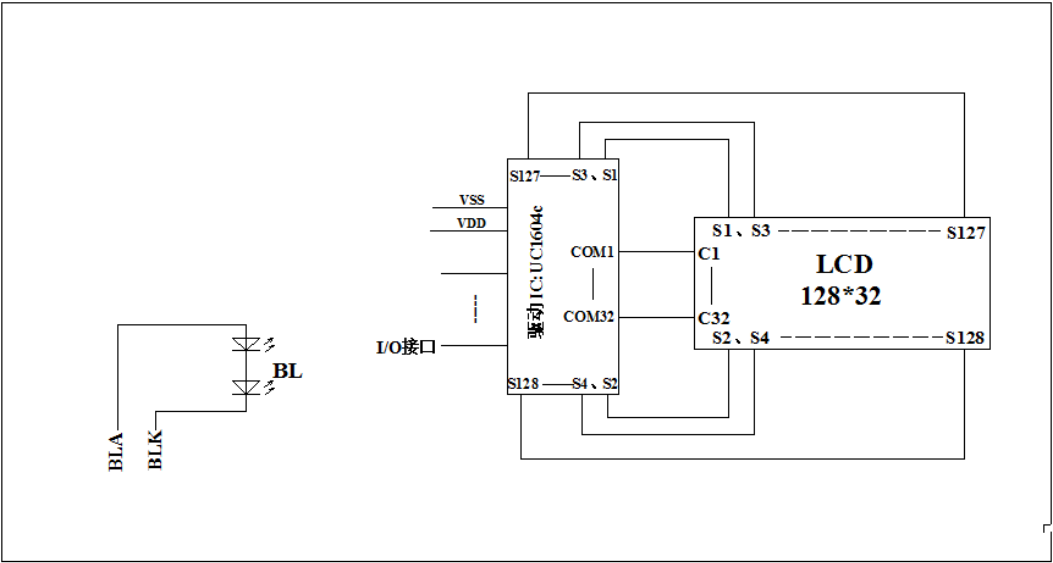
图 2：JLX128G-908 图像点阵型液晶模块的电路框图
