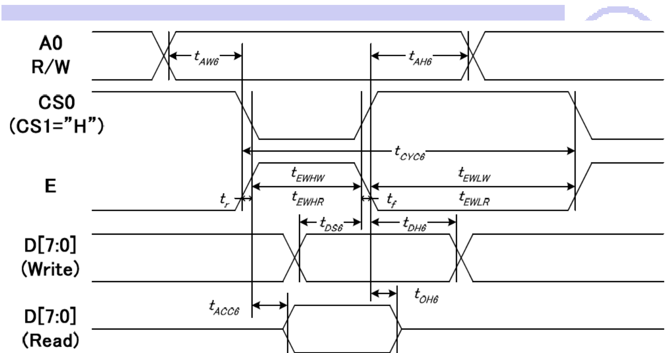
图 5. 从 CPU 写到 ST7525I（Writing Data from CPU to ST7525I）
