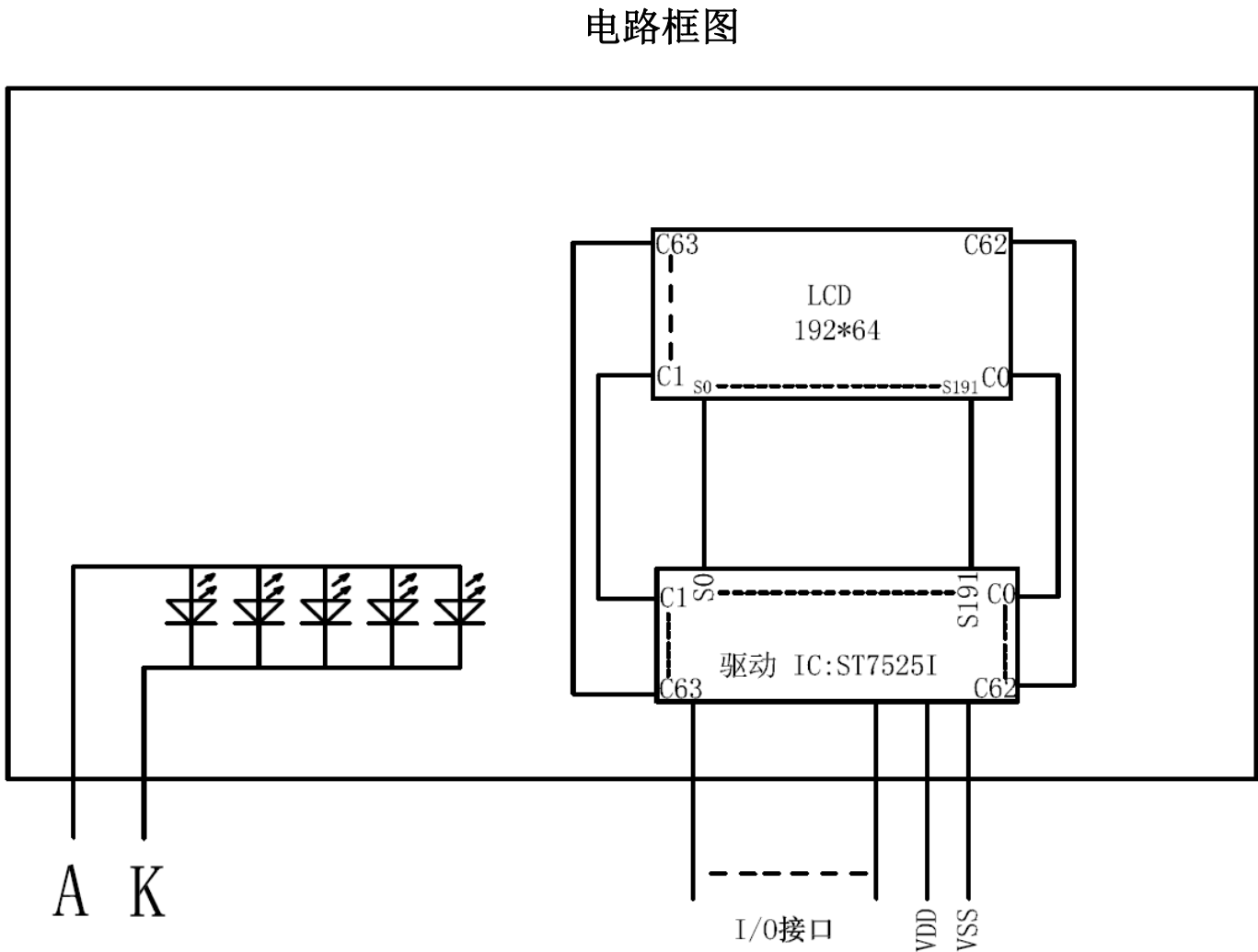
图 2:JLX19264G-90102 图像点阵型液晶模块的电路框图
