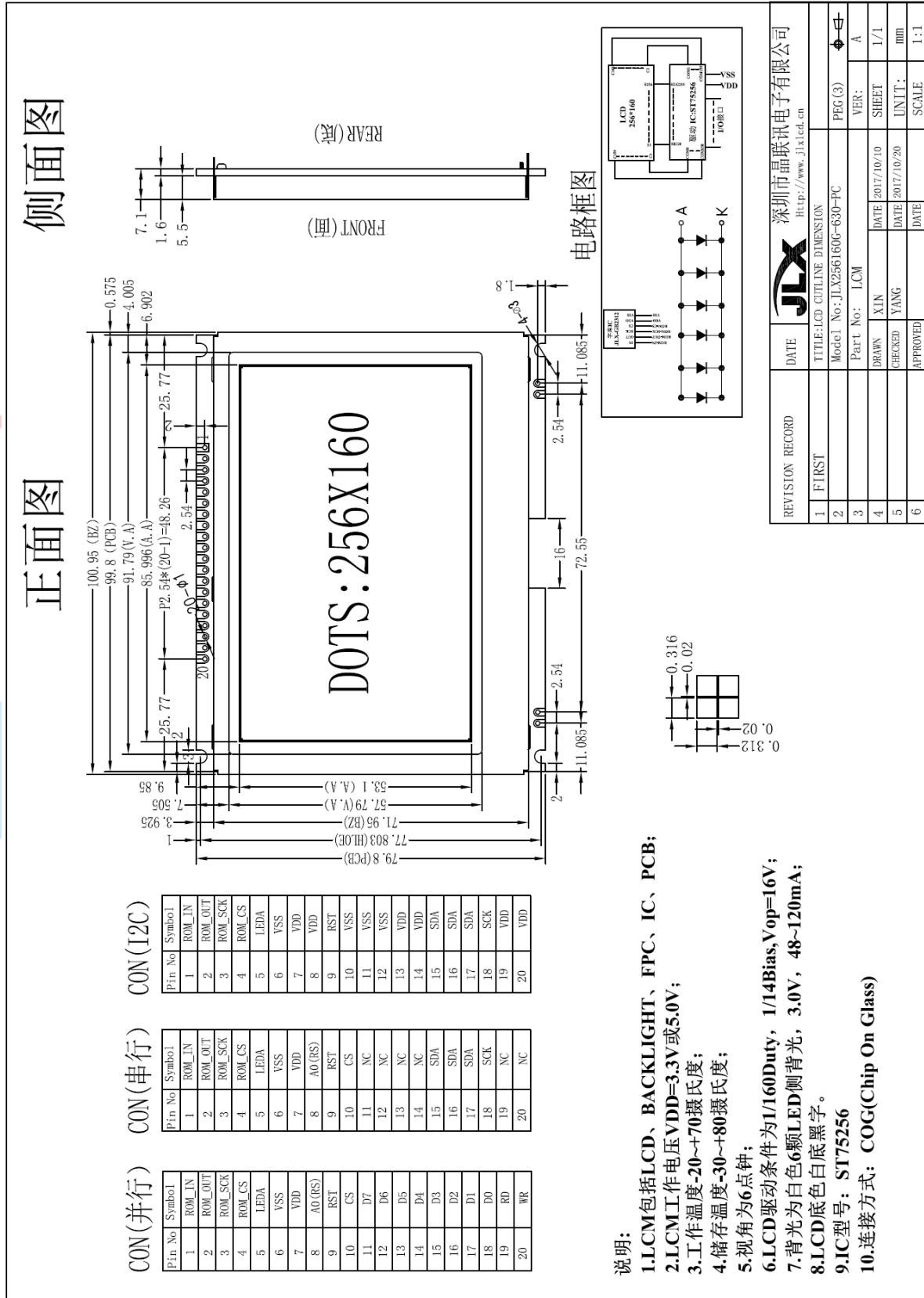
图 1. 外形尺寸
