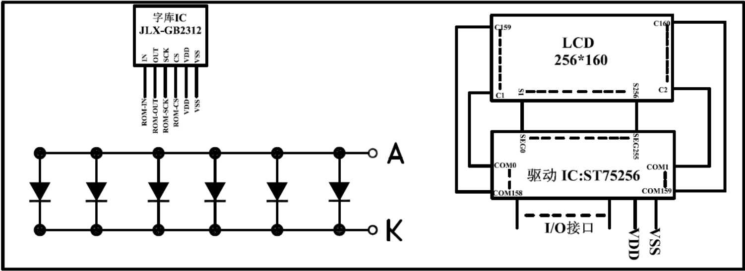
图 2：JLX256160G-630-PC 电路框图
