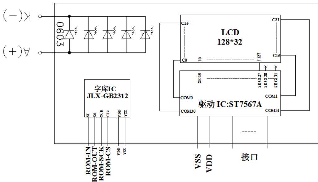
图 2: 电路框图
