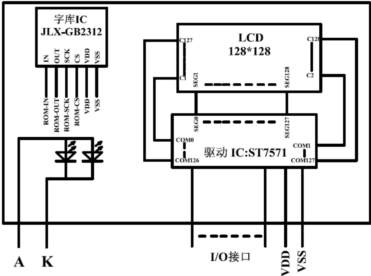
图 2: JLX128128G-560 图像点阵型液晶模块的电路框图
