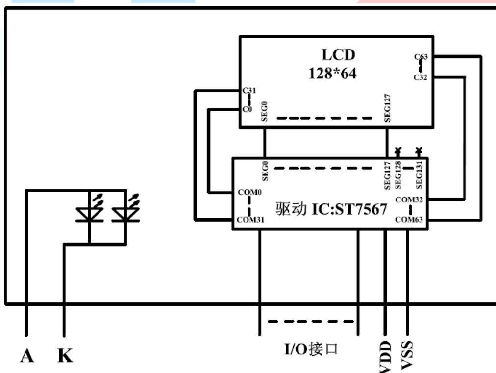
图 2: JLX12864G-290-PN 图像点阵型液晶模块的电路框图
