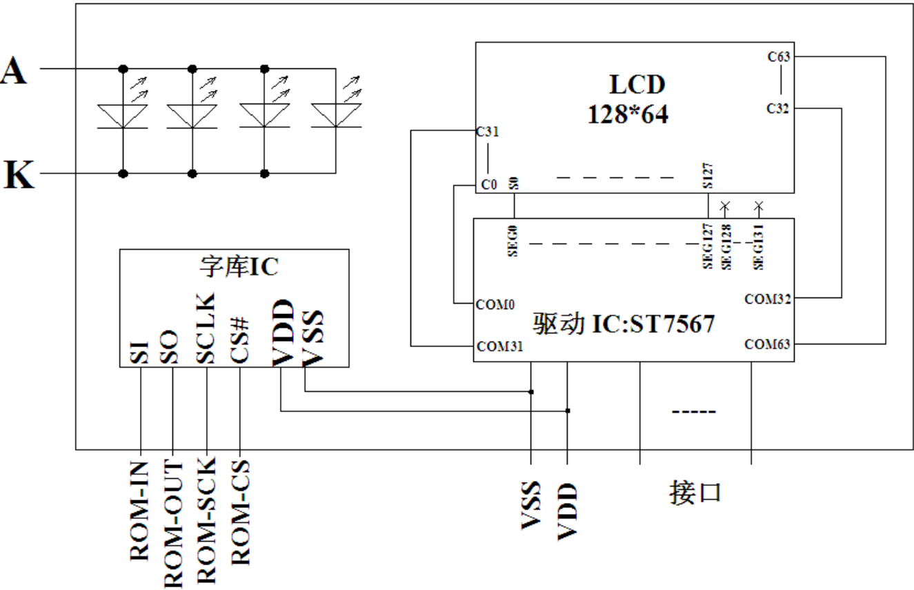
图 2: 电路框图
